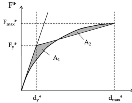
Figura C7.3.3- Bilinearizzazione equivalente
