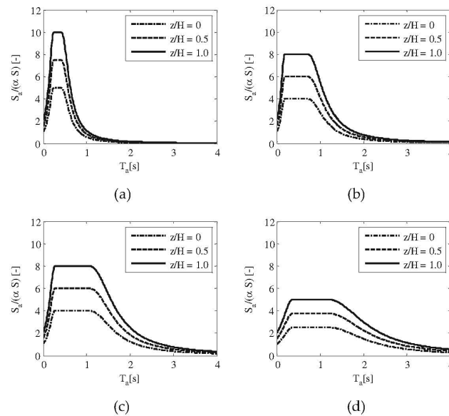
Figura C7.2.4 - Accelerazione massima, normalizzata rispetto ad \alpha S , per i seguenti valori di T_i : (a) T_i = 0,3 s, (b) T_i = 0,6 s, (c) T_i = 0,9 s, (d) T_i = 1,2 s.
