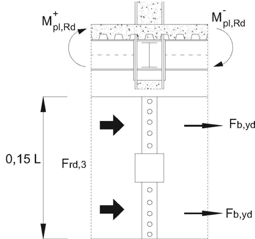
Figura C7.6.5 - Meccanismo 3 – Connettori a taglio sulle travi secondarie
